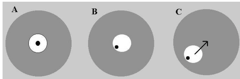
Figura 3: Aspetto di una stella sfuocata al centro del campo con ottica collimata (A), con ottica non collimata (B) e dove posizionarla e come muoverla per collimarla (C). Il cerchio grigio scuro è sempre il campo inquadrato dall'oculare, nelle tre figure A B e C.
