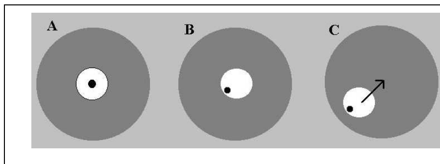
Figura 3: Aspetto di una stella sfocata al centro del campo con ottica collimata (A), con ottica non collimata (B) e dove posizionarla e come muoverla per collimarla (C). Il cerchio grigio scuro è sempre il campo inquadrato dall'oculare, nelle tre figure A B e C.
