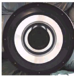
Figura 2: Aspetto degli specchi NON collimati
